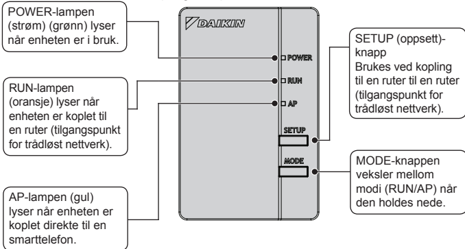
Tilkoplingsadapter for trådløst nettverk
